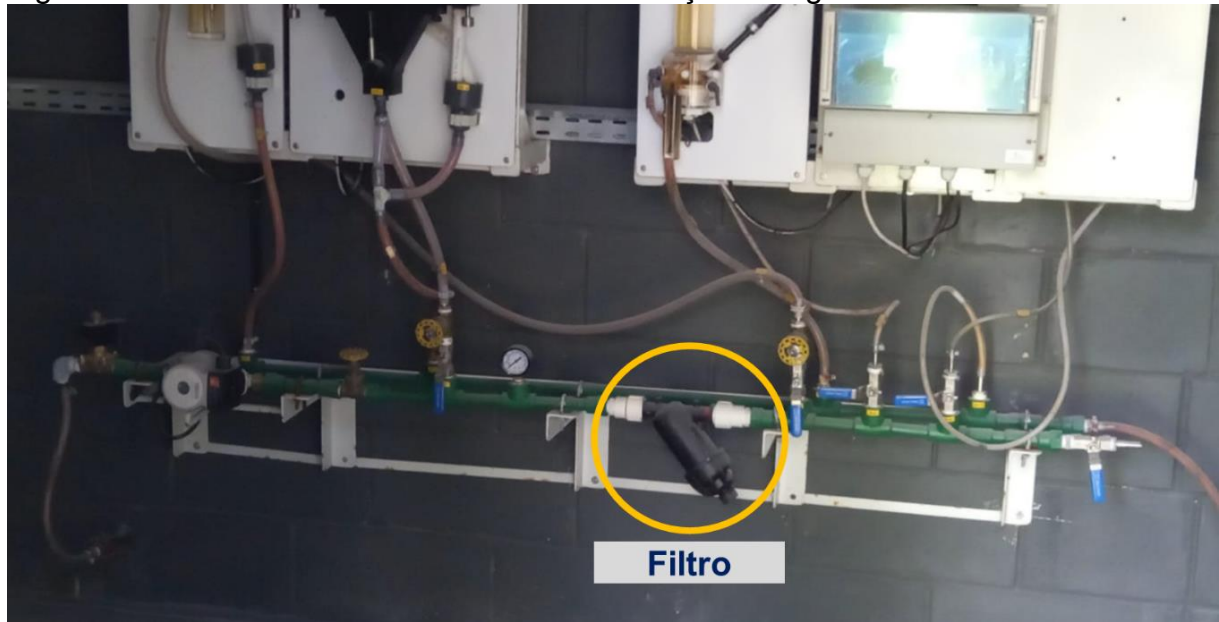
Figura 18 – Filtro instalado na linha de alimentação de água do SMO.
