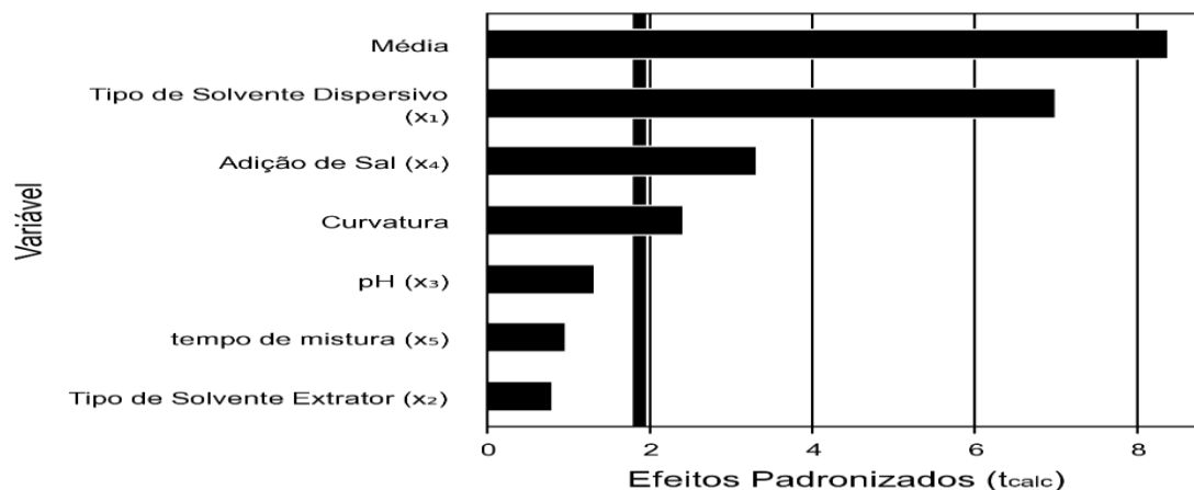
Figura 19 - Diagrama de Pareto dos Efeitos Padronizados PB12 – BPS
