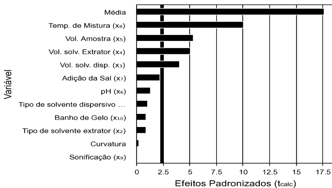
Figura 12 - Diagrama de Pareto dos Efeitos Padronizados PB16 - BPA
