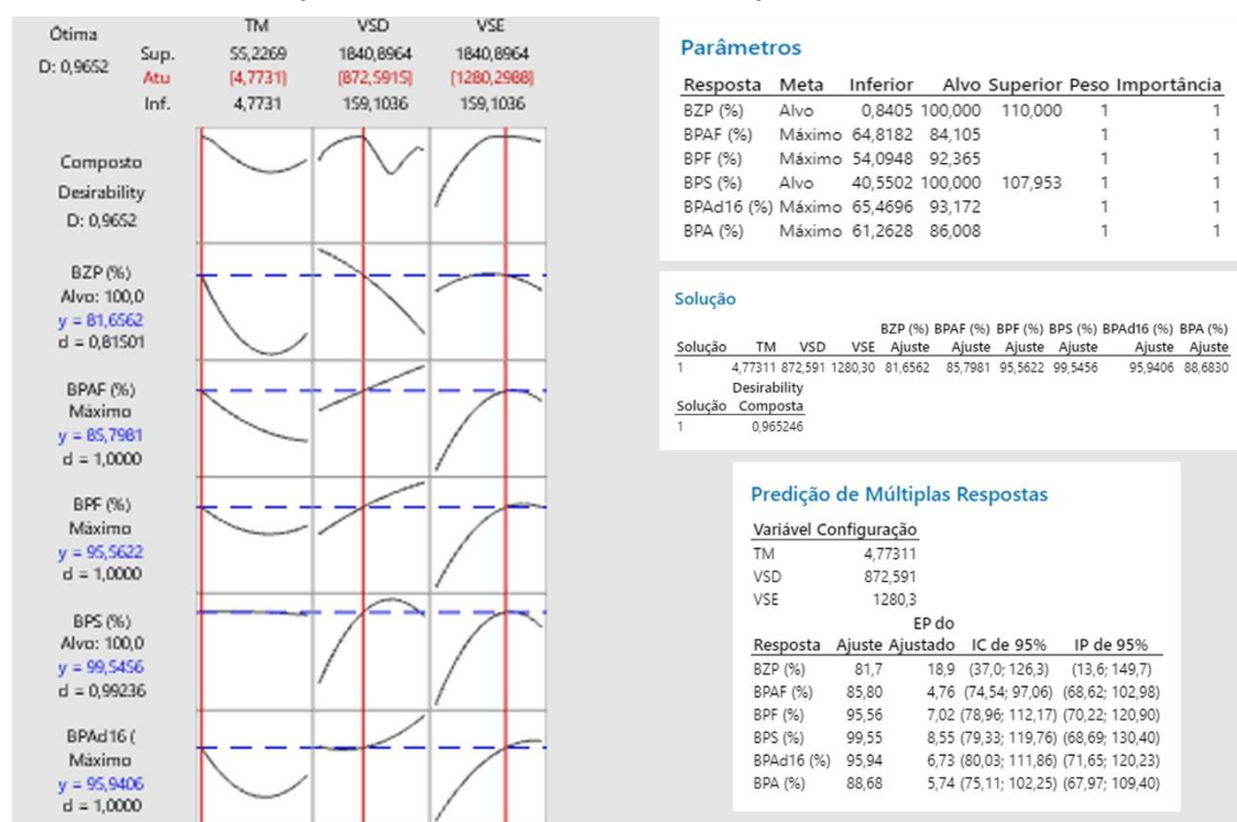
Figura 25 - Otimização da Resposta através da função desejabilidade
