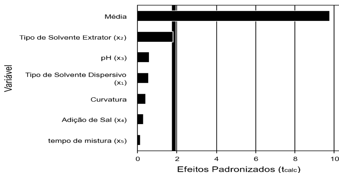
Figura 21 - Diagrama de Pareto dos Efeitos Padronizados PB12 – BZP
