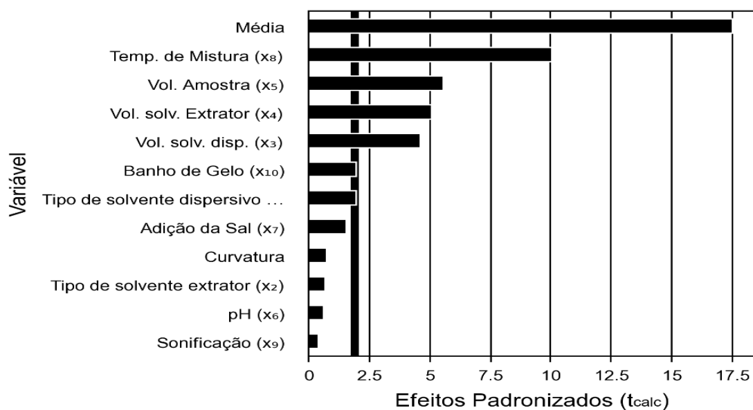
Figura 13 - Diagrama de Pareto dos Efeitos Padronizados PB16 - BPA d16
