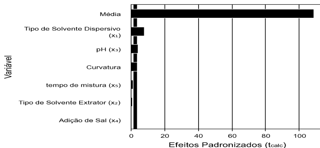
Figura 20 - Diagrama de Pareto dos Efeitos Padronizados PB12 – BPAF
