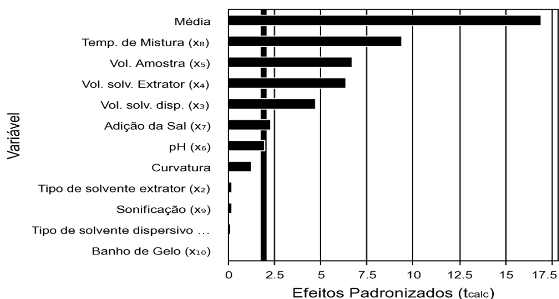
Figura 15 - Diagrama de Pareto dos Efeitos Padronizados PB16 - BPF
