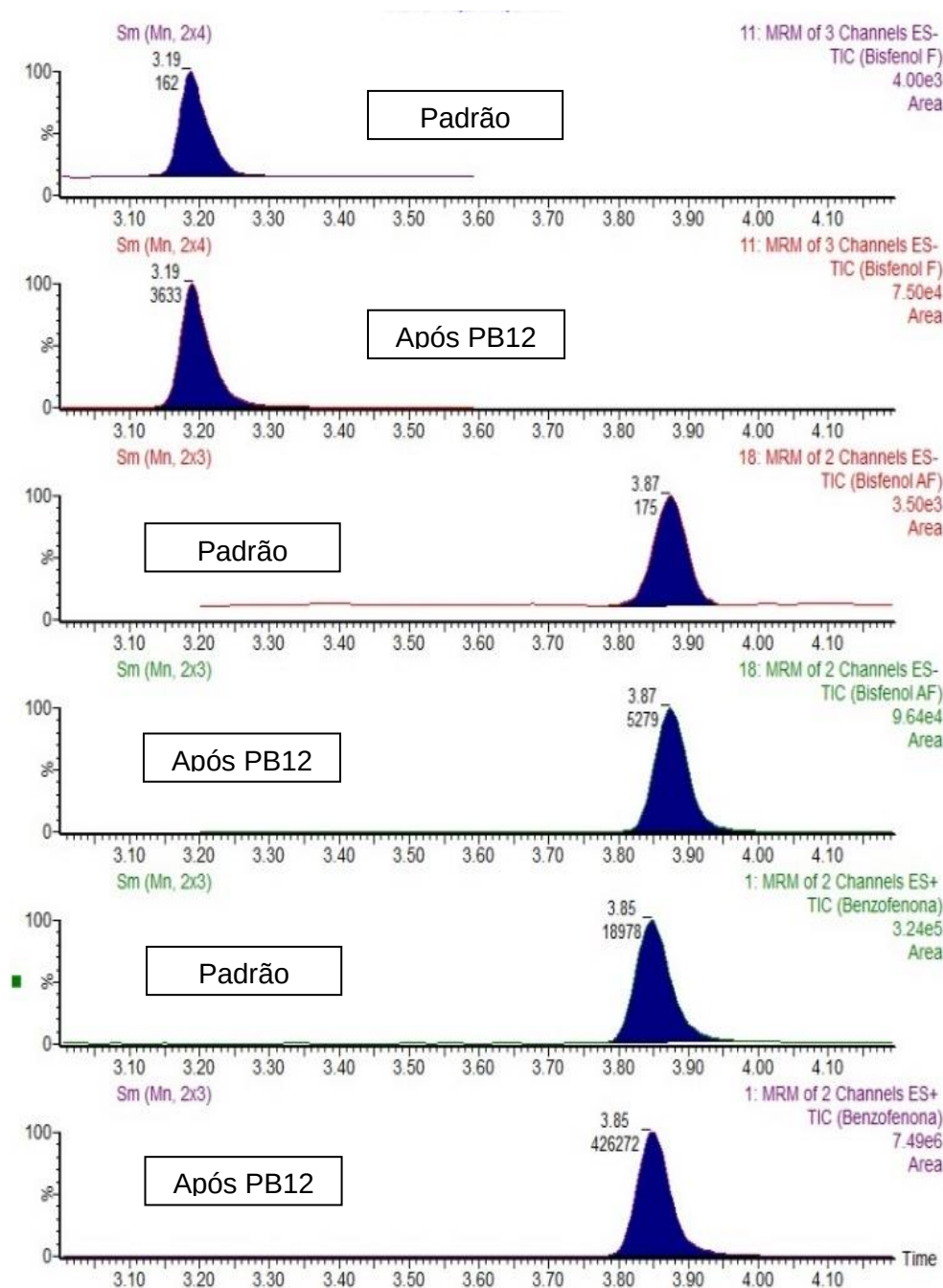
Figura 23 - Cromatograma: Padrão (BPF, BPS e BZP) versus melhores condições alcançadas pela DLLME com base no PB12.
