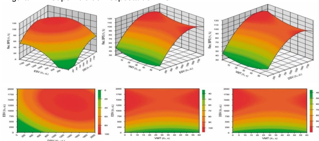
Figura 24 - Superfície de Resposta do BPS.
