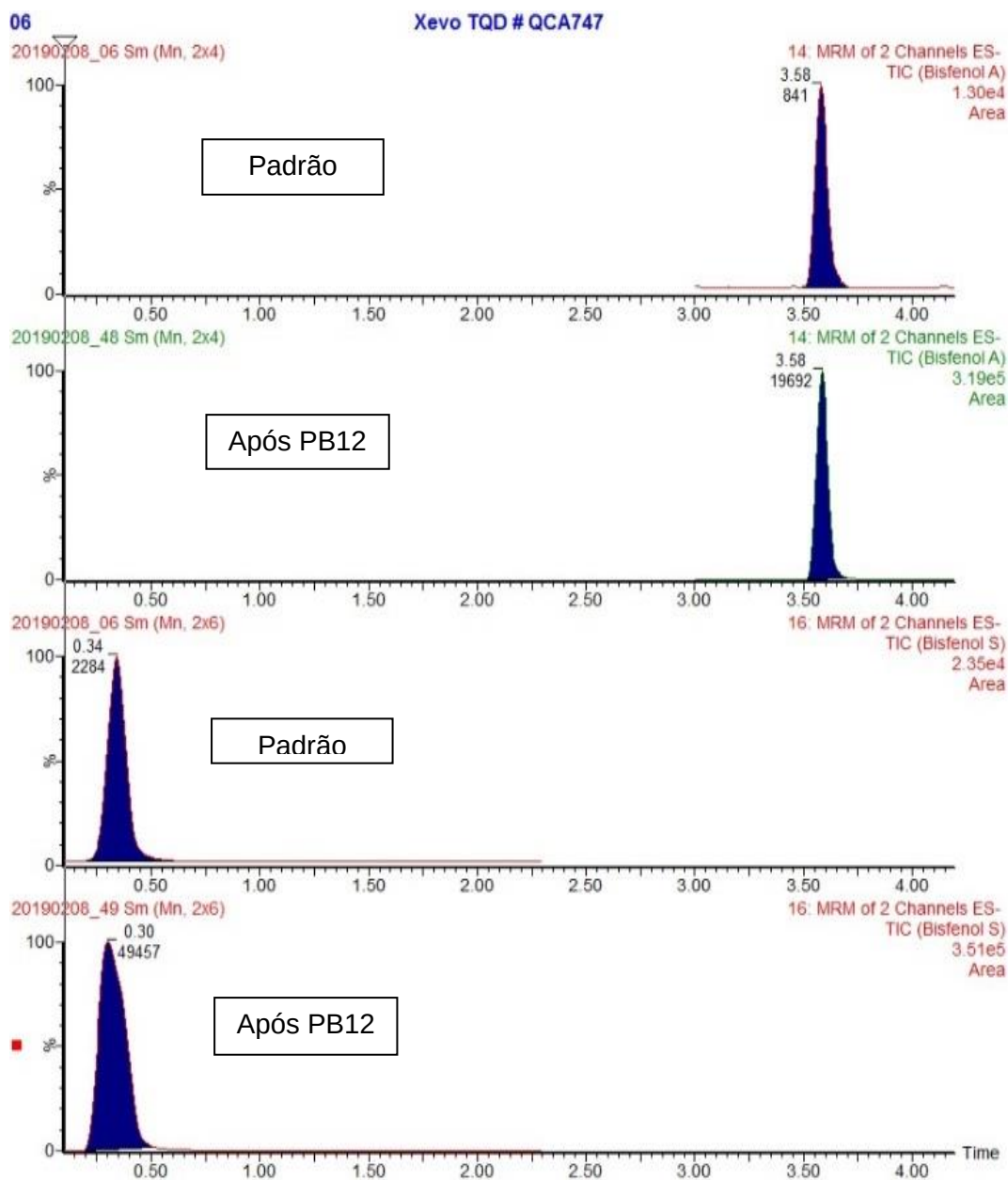
Figura 22 - Cromatograma: Padrão (BPA e BPS) versus melhores condições alcançadas pela MELLD com base no PB12.
