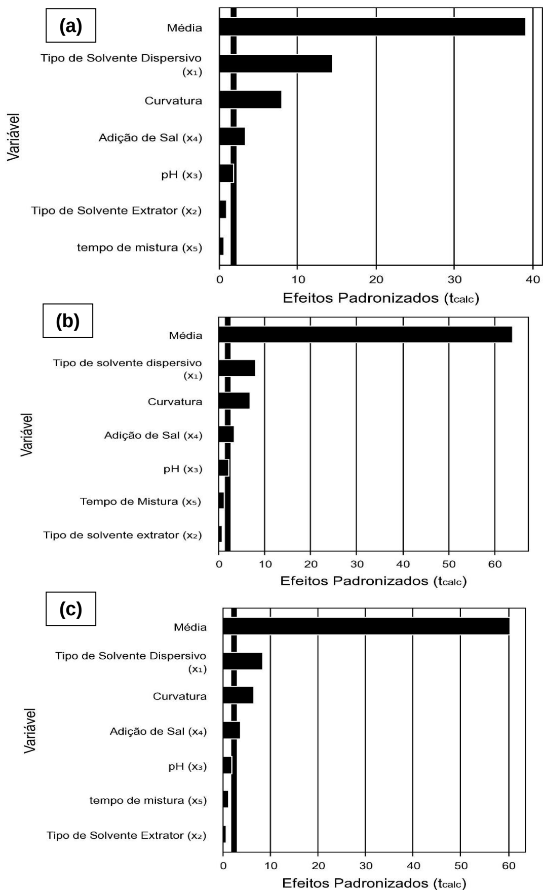
Figura 18 - Diagrama de Pareto dos Efeitos Padronizados PB12 – BPA (a), BPAd 16 (b) e BPF (c)
