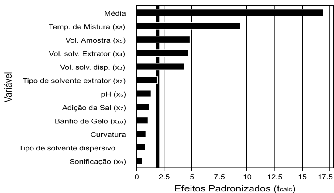
Figura 16 - Diagrama de Pareto dos Efeitos Padronizados PB16 - BPAF
