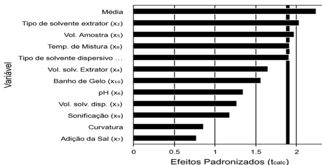
Figura 17 - Diagrama de Pareto dos Efeitos Padronizados PB16 - BZP
