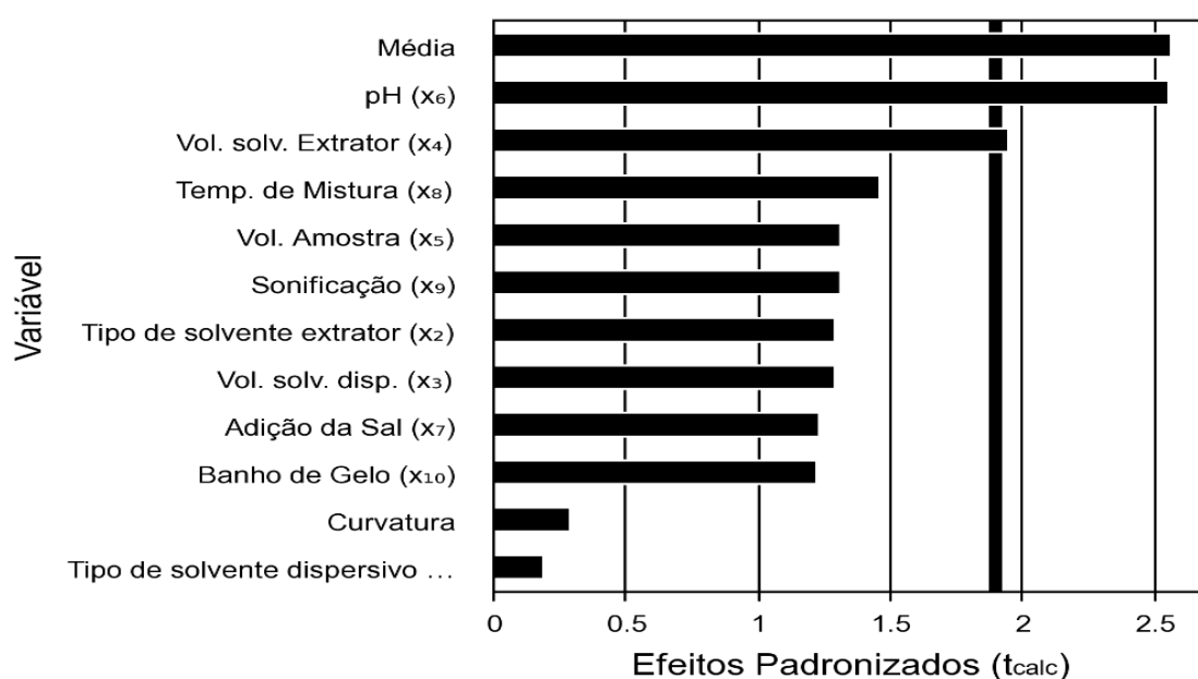
Figura 14 - Diagrama de Pareto dos Efeitos Padronizados PB16 - BPS
