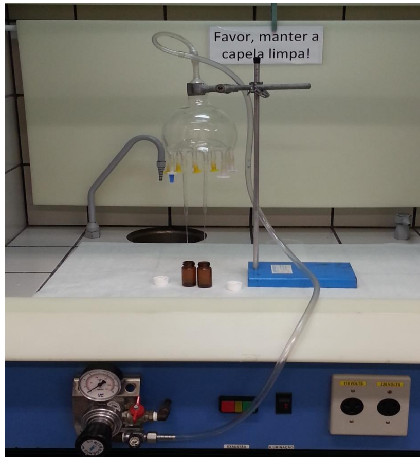
Figura 23 - Foto do aparato de secagem com fluxo de nitrogênio
