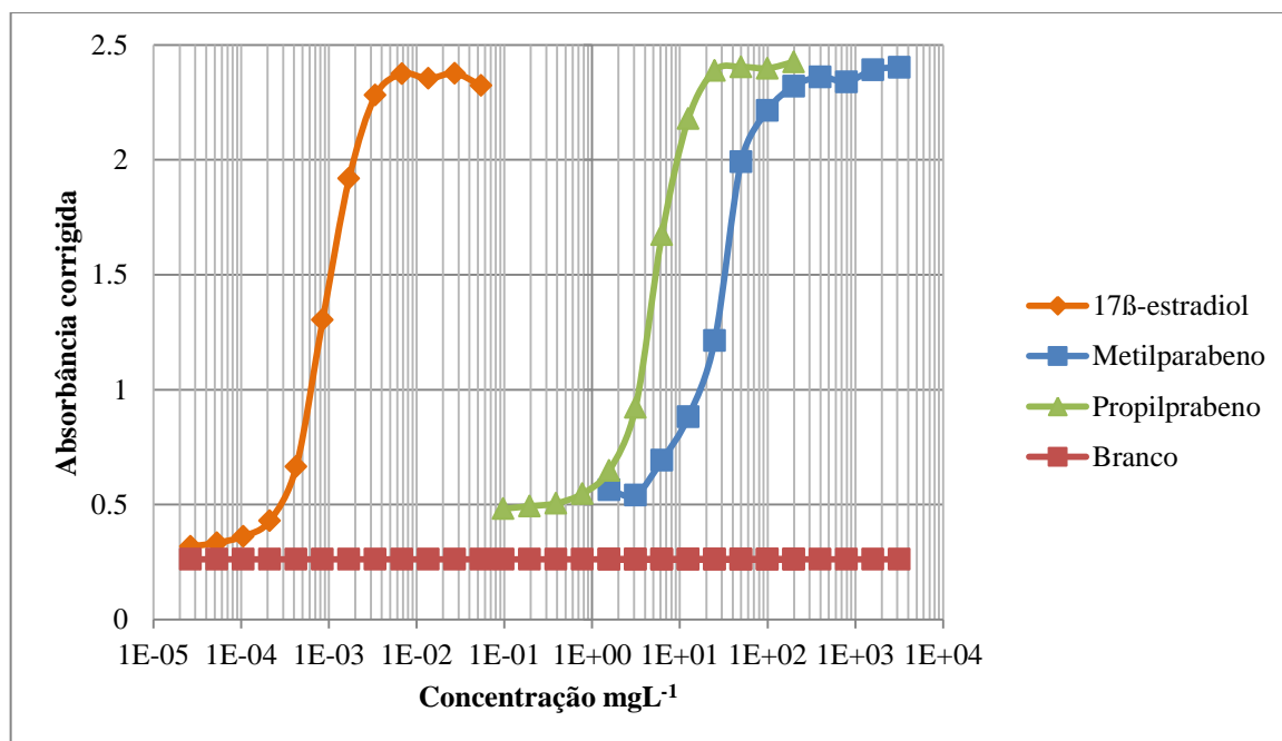
Figura 32 - Curva dose resposta no ensaio YES dos parabenos e do 17 \beta -estradiol
