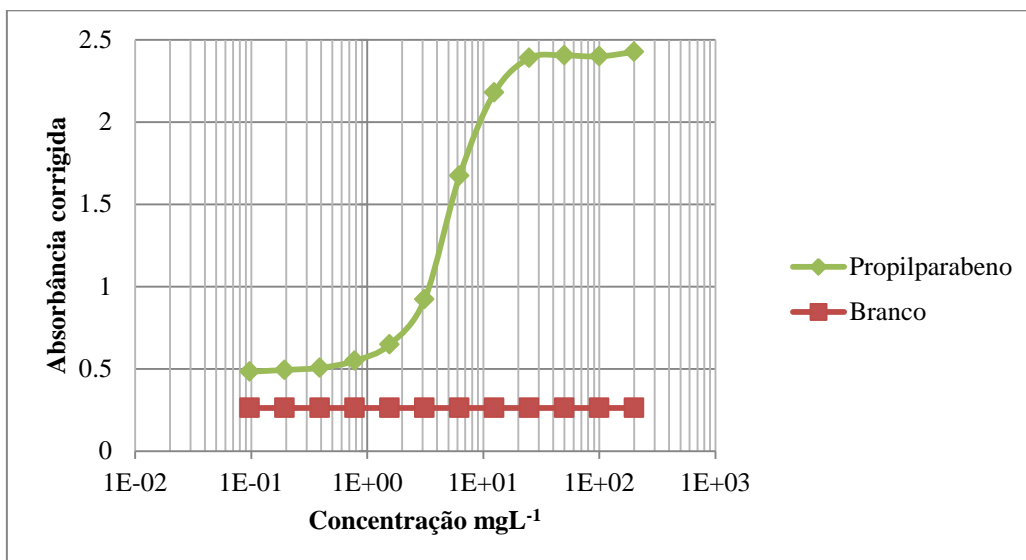
Figura 31 - Curva dose-resposta do parabeno Propilparabeno obtida na faixa de 200 \text{mgL}^{-1} a 0,098 \text{mgL}^{-1} .
