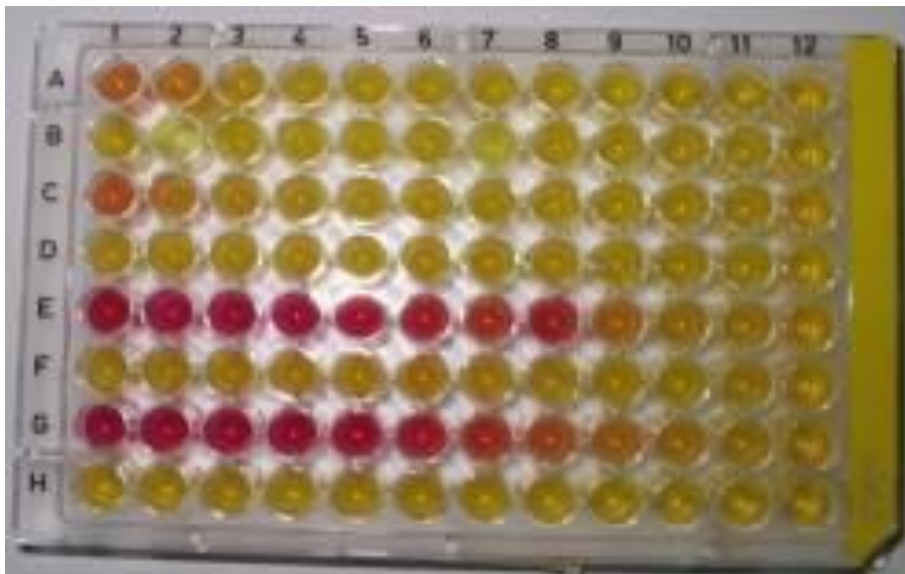
Figura 2 - Placa de 96 poços contendo substâncias estrogênicas na ordem de mais concentrado para menos concentrado.
