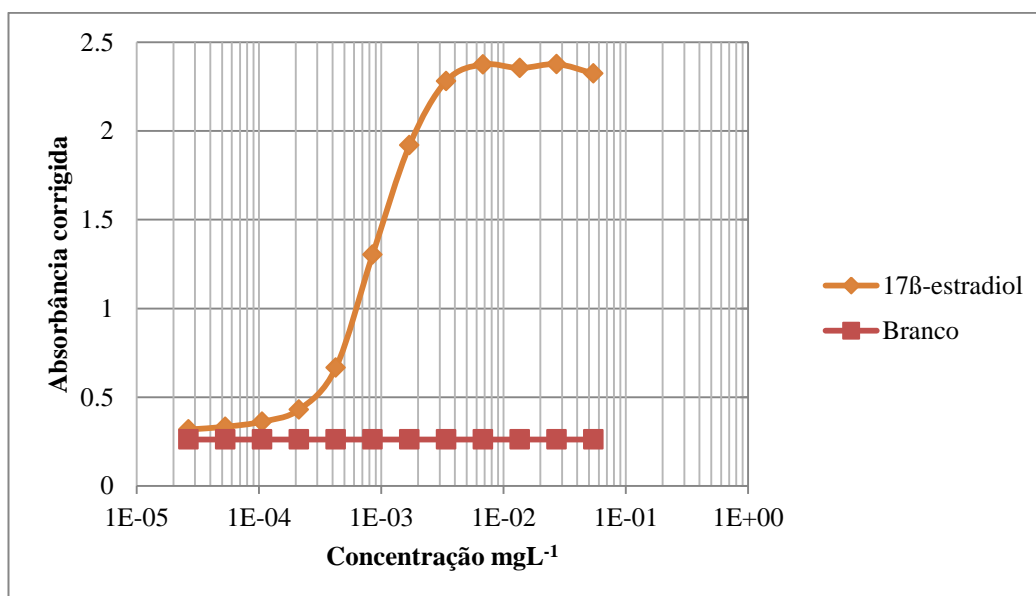
Figura 29 - Curva dose resposta do 17 \beta -estradiol obtida na faixa de concentração de 5,44 \times 10^{-2} \text{ mgL}^{-1} a 2,66 \times 10^{-5} \text{ mgL}^{-1}
