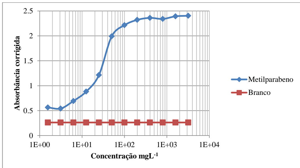
Figura 30 - Curva dose-resposta do parabeno Metilparabeno obtida na faixa de concentração de 3200 \text{ mgL}^{-1} a 1,56 \text{ mgL}^{-1} .
