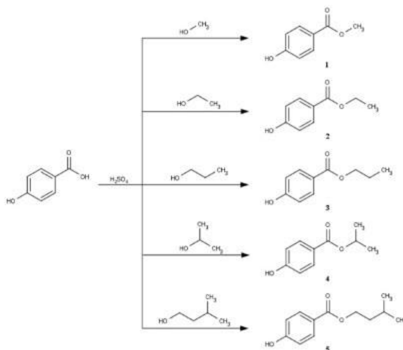
Figura 7 - Esquema sintético das reações realizadas para obtenção dos parabenos 1-5
