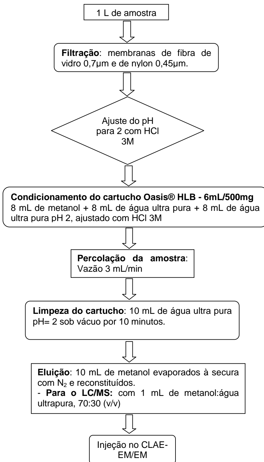
Figura 25 - Fluxograma para a determinação dos parabenos por CLAE-EM/EM das amostras coletadas no Rio Maracanã.
