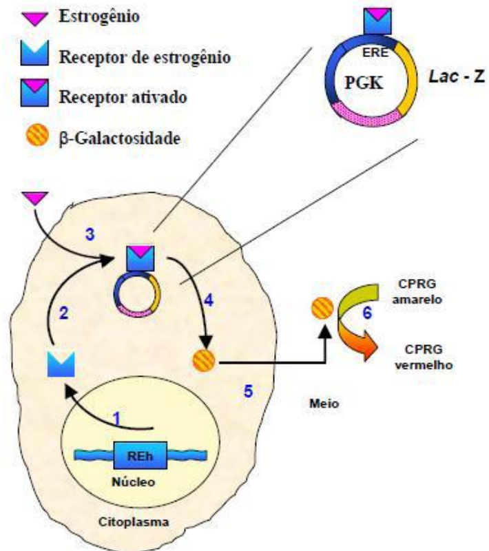
Figura 1 - Esquema do sistema de expressão do composto estrogênio-induzível presente na levedura Saccharomyces cerevisiae
